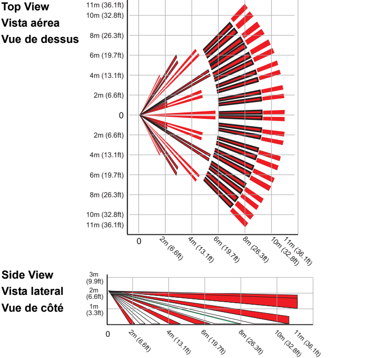
Figure/Figura 2 DG75+ Pet Array Beam Pattern / Estructura de Haces / Diagramme de faisceau
